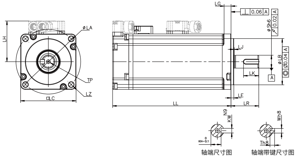
MS1H1（Vn=3000rpm，Vmax=6000rpm）系列外形尺寸图（单位：mm）
