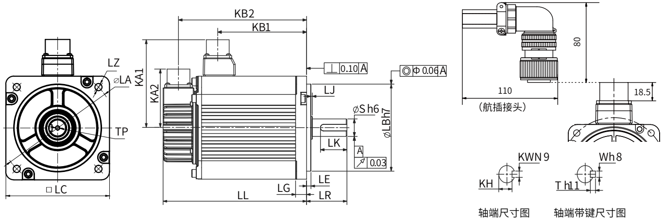
MS1H3 (Vn=1500rpm, Vmax=3000rpm) 系列外形尺寸图 (单位: mm)
