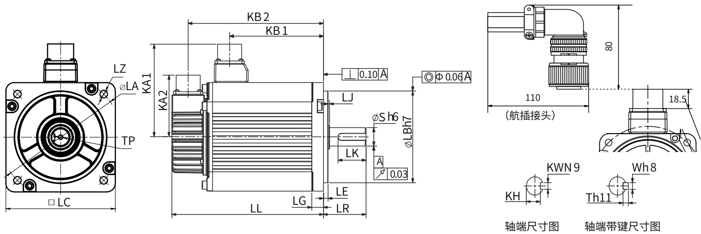
MS1H2 (Vn=3000rpm, Vmax=6000/5000rpm) 系列外形尺寸图 (单位: mm)
