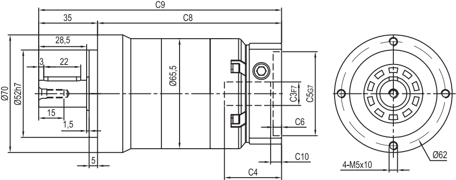
输出端 / OUTPUT
