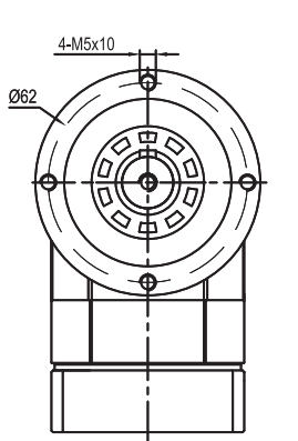
输出端 / OUTPUT
