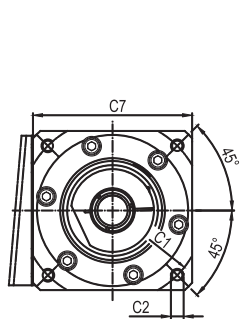
输入端/ INPUT
