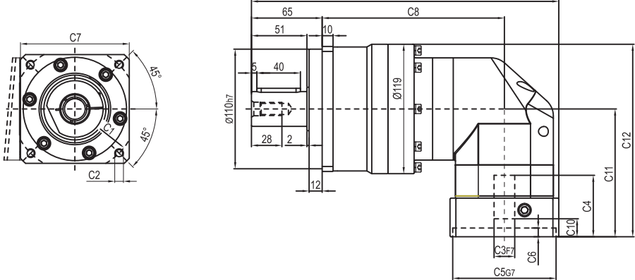
输入端 / INPUT
