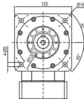
输出端 / OUTPUT
