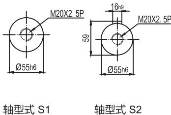
轴型式 S1 轴型式 S2
