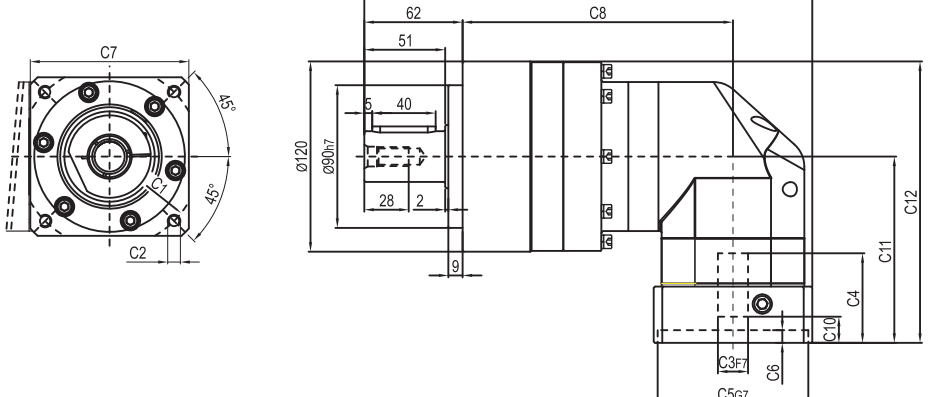
输入端 / INPUT
