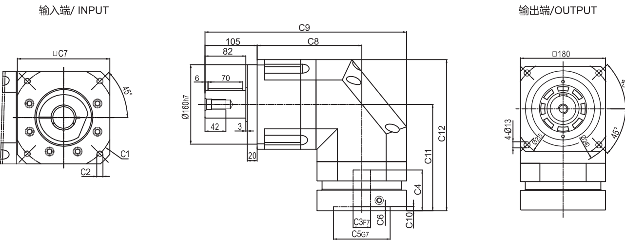
FABR-180D-L2
