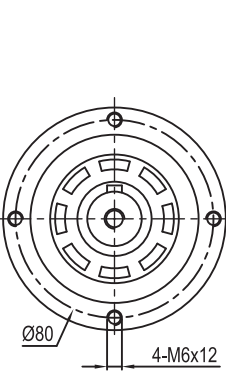
输出端 / OUTPUT
