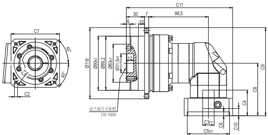
输入端/ INPUT
