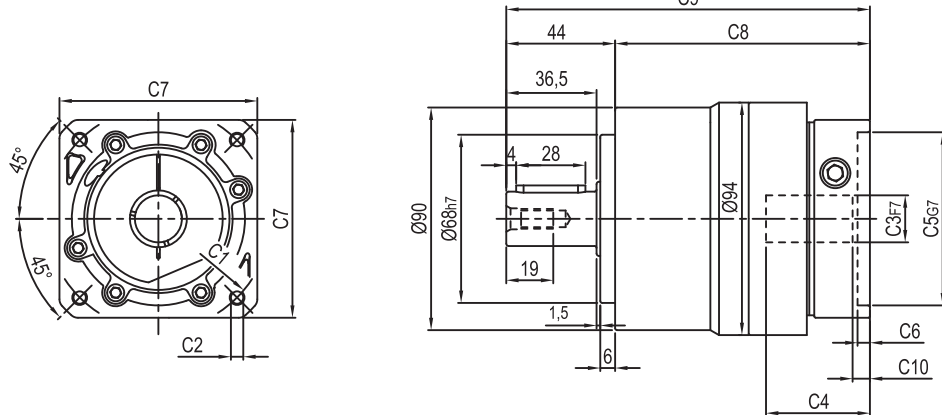
输入端 / INPUT
