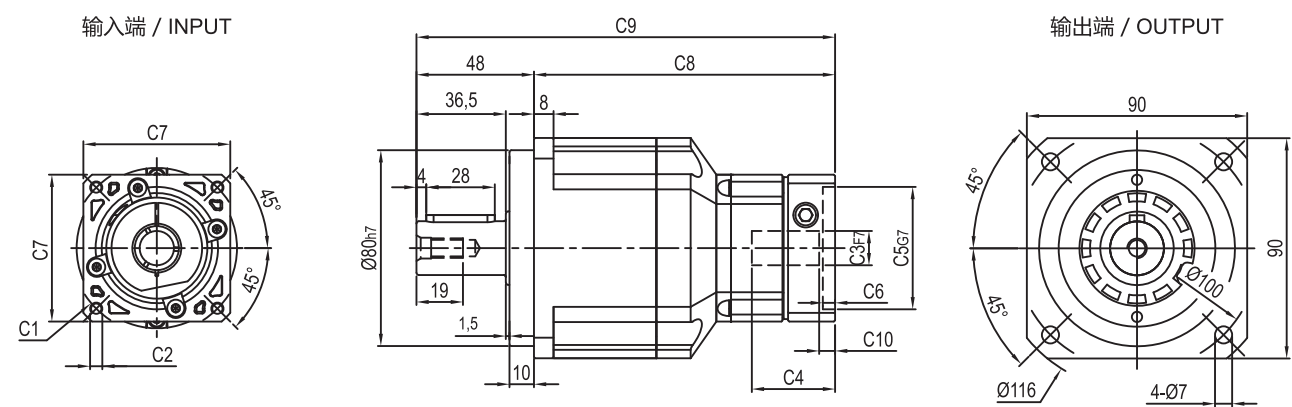
FAB-090D(M1)-L2
