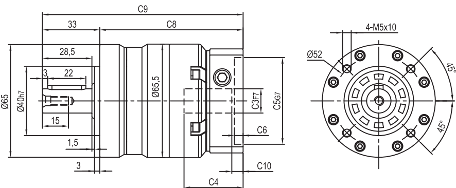
输出端/ OUTPUT
