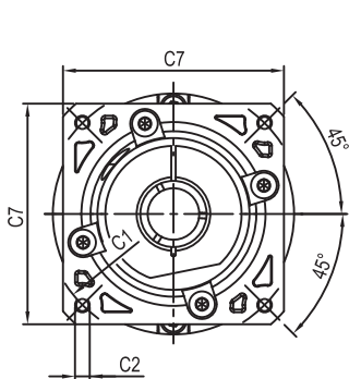
输入端/INPUT
