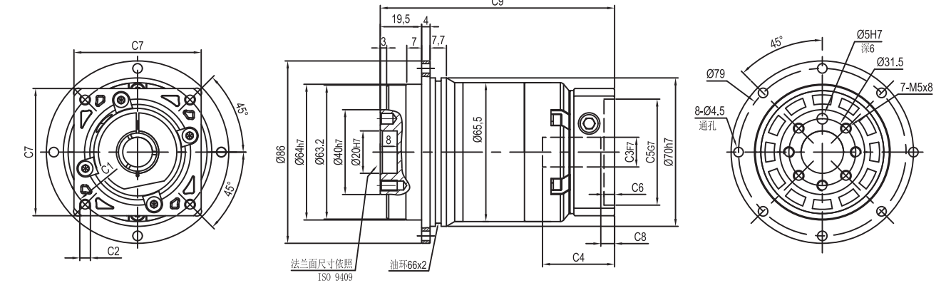
输入端/ INPUT
