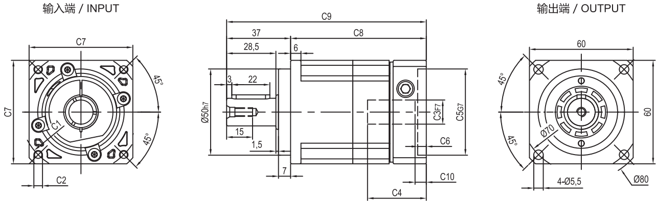
FAB-060D(M1)-L1
