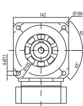
输出端 / OUTPUT
