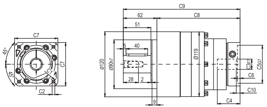
输入端 / INPUT
