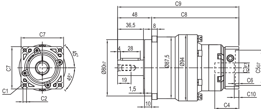
输入端 / INPUT
