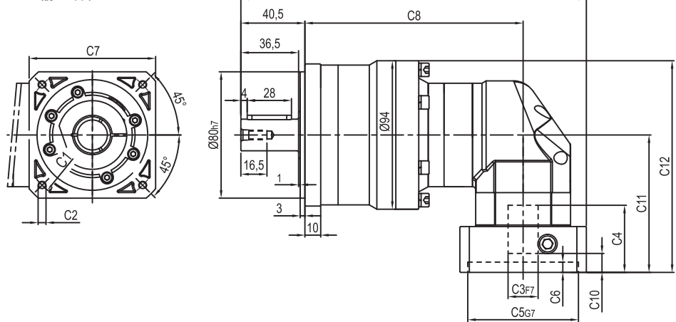
输入端 / INPUT
