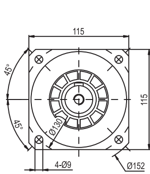
输出端/ OUTPUT
