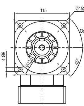
输出端 / OUTPUT
