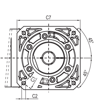
输入端/INPUT
