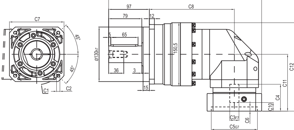
输入端 / INPUT
