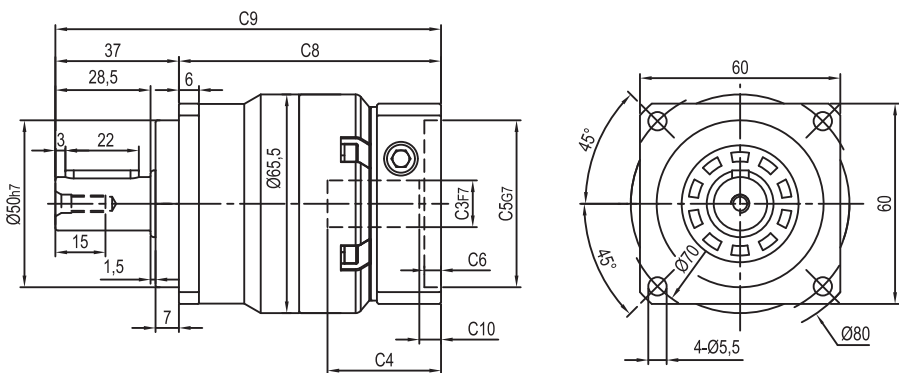
输出端 / OUTPUT
