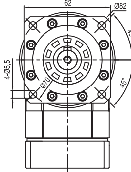
输出端 / OUTPUT
