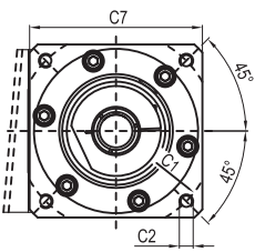
输入端/ INPUT
