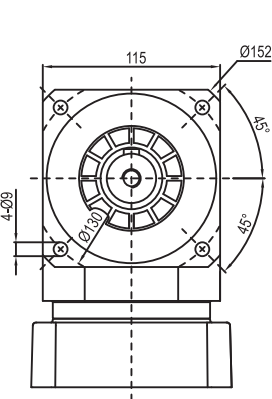
输出端 / OUTPUT
