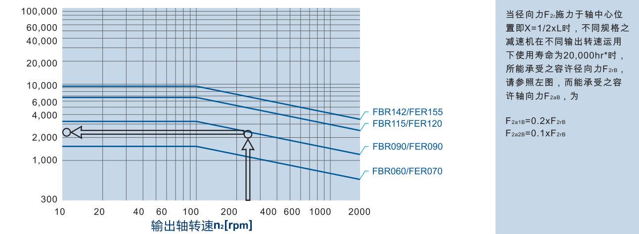
容许径向力 F 2rB [N] 施力于轴中心位置
