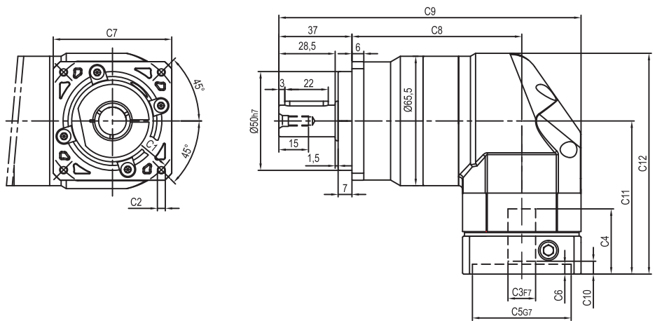
输入端 / INPUT
