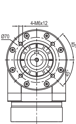
输出端/ OUTPUT
