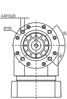
输出端/ OUTPUT
