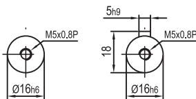
轴型式 S1
