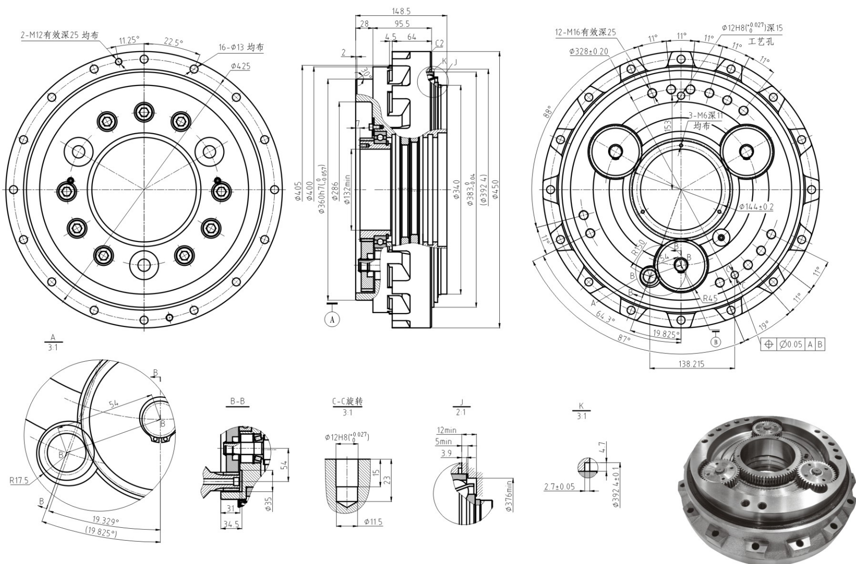
■ BX320CA 输出轴螺栓紧固型外形尺寸图
