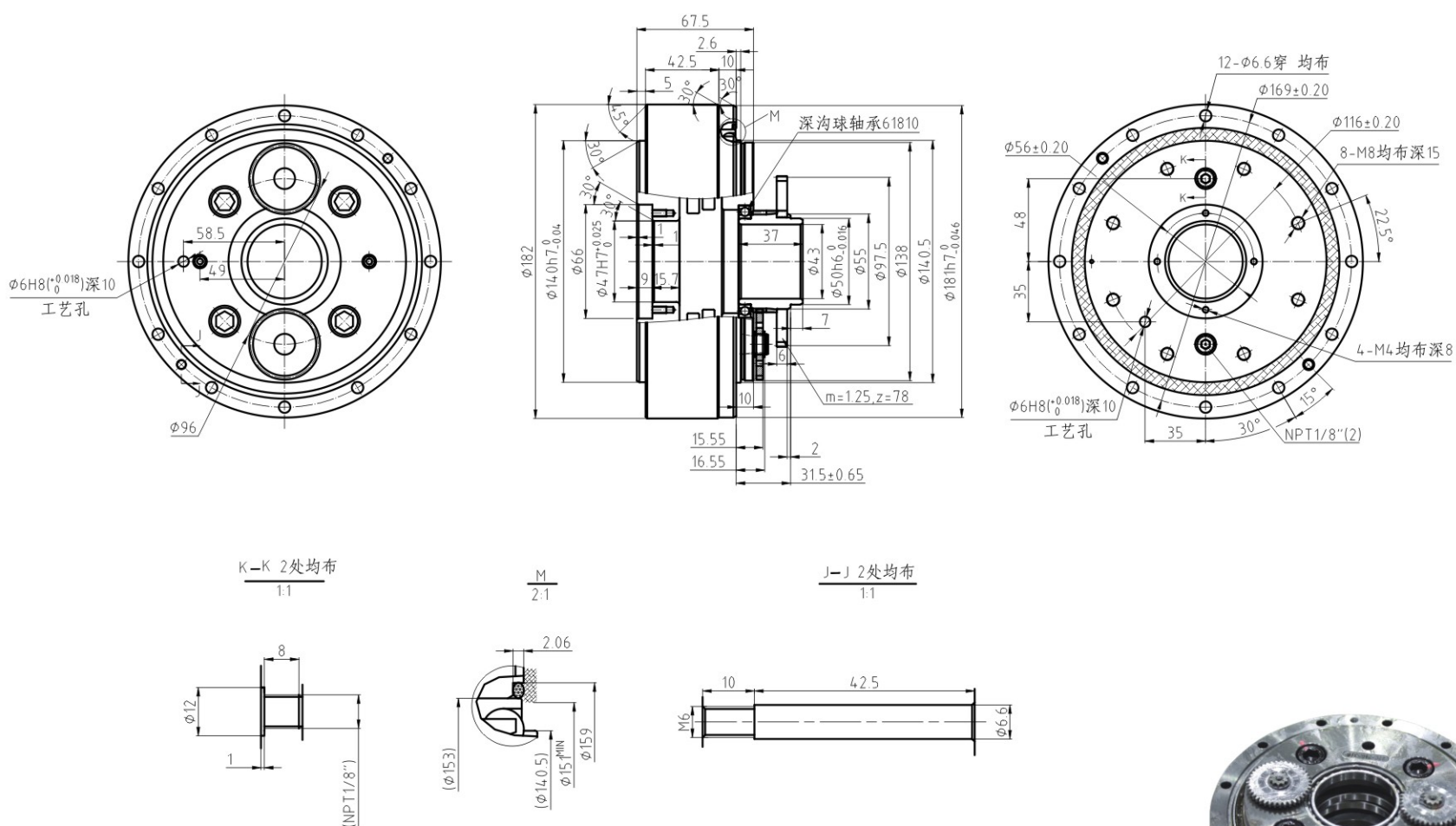
■ BX27C 输出轴螺栓紧固型外形尺寸图
