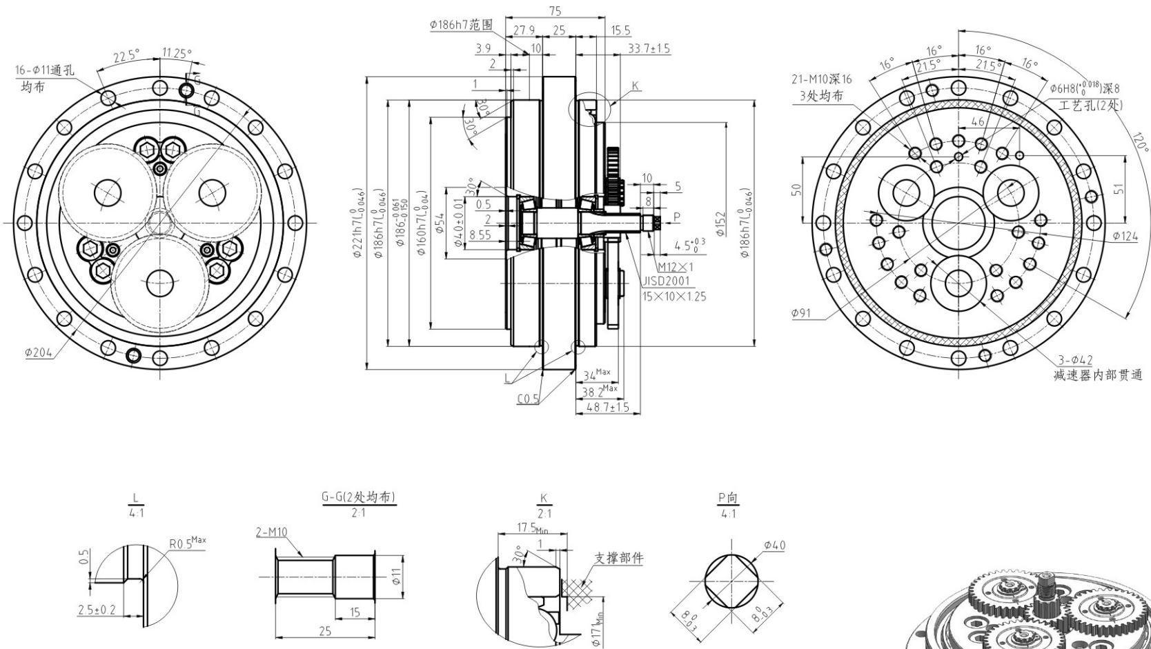
BX125N/i1111T 外形尺寸图
