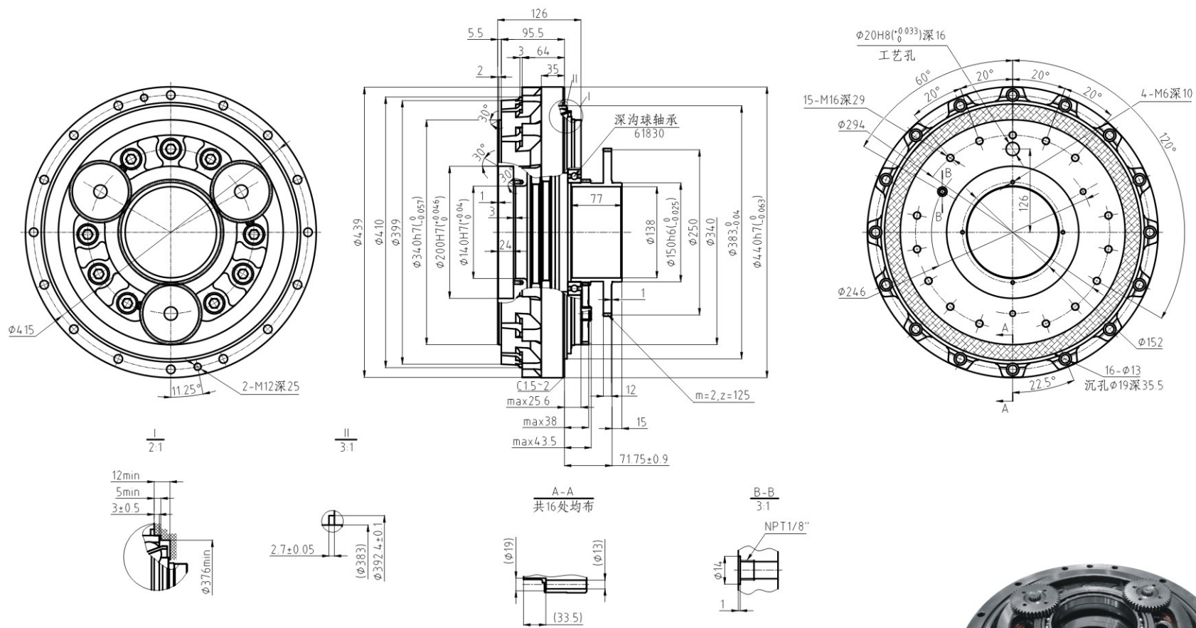
■ BX320C 输出轴螺栓紧固型外形尺寸图
