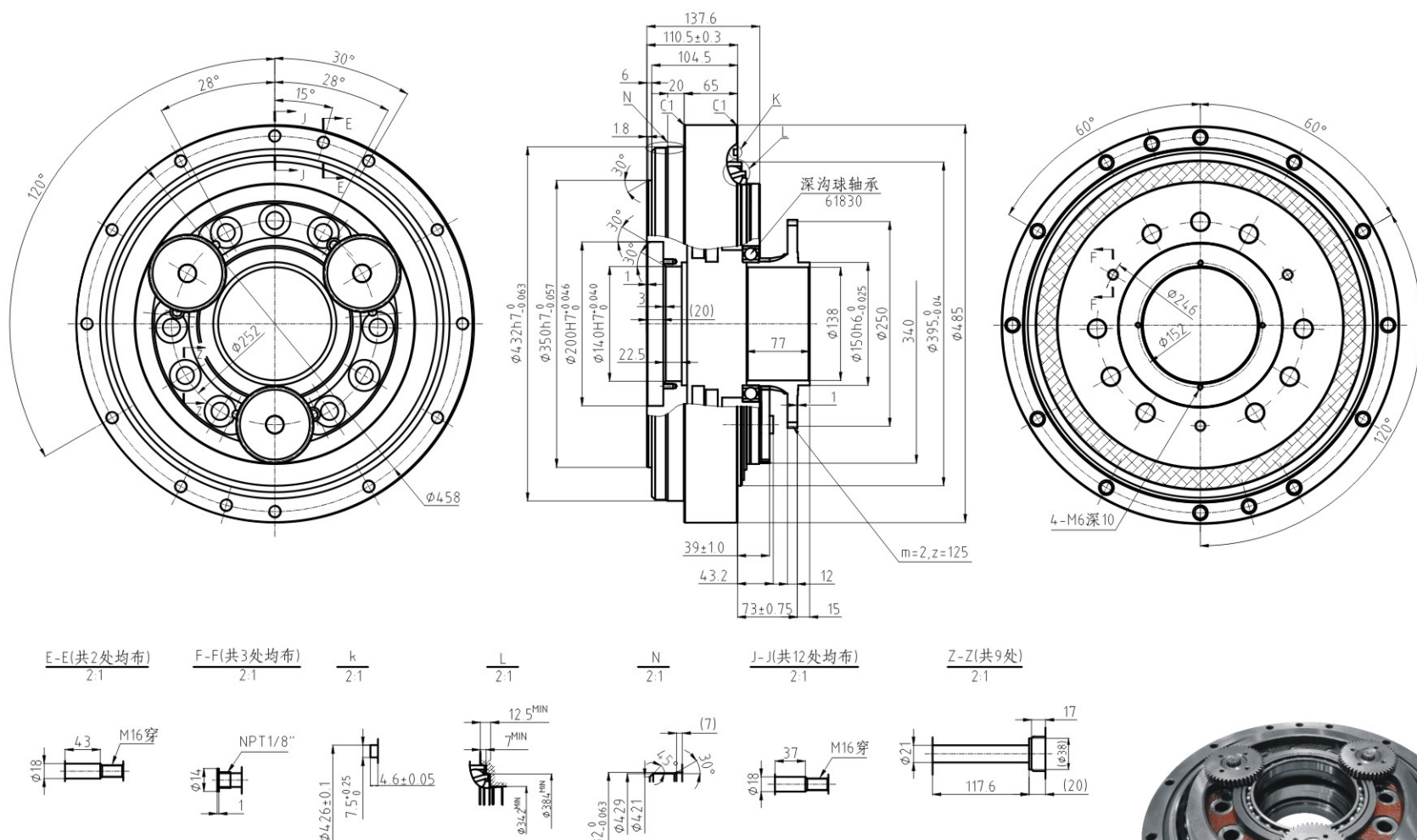
■ BX400C 输出轴螺栓紧固型外形尺寸图
