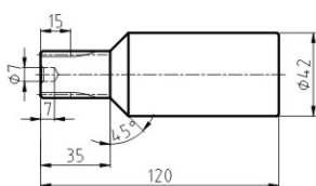
输入齿轮 型式A
