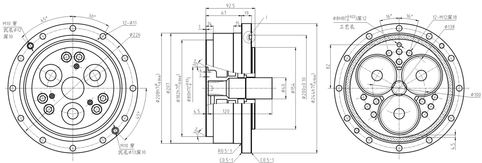
■ BX110E 输出轴螺栓紧固型外形尺寸图
