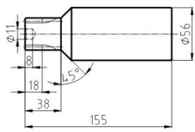
输入齿轮 型式A
