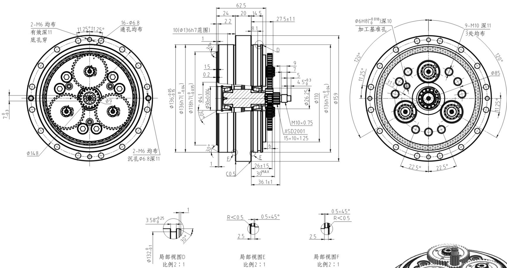
BX42N/i81T 外形尺寸图
