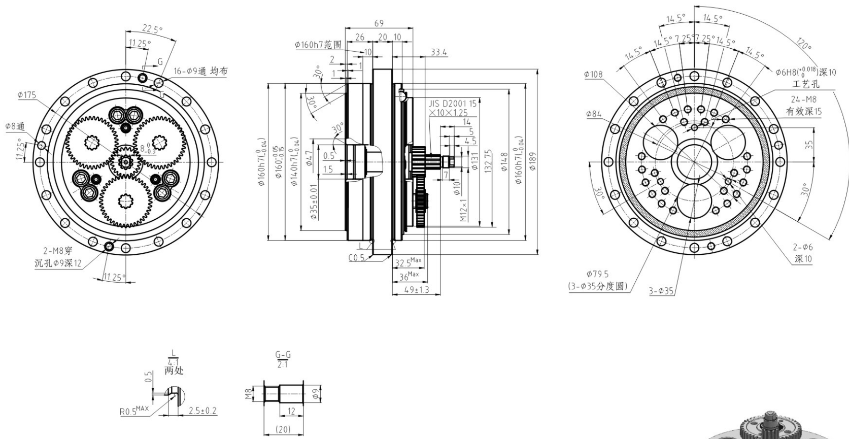
BX80N/i75.54T 外形尺寸图
