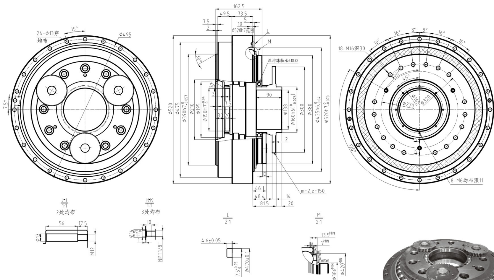
■ BX500C 输出轴螺栓紧固型外形尺寸图
