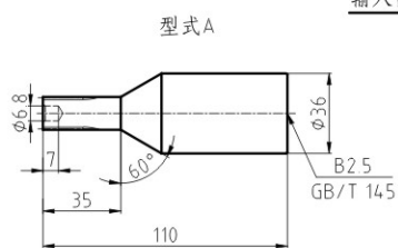
输入齿轮
