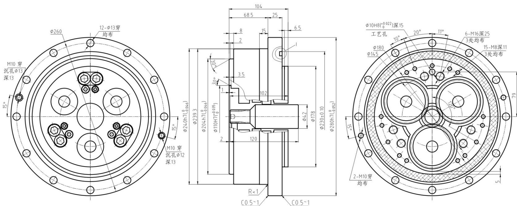
输入齿轮 型式A
