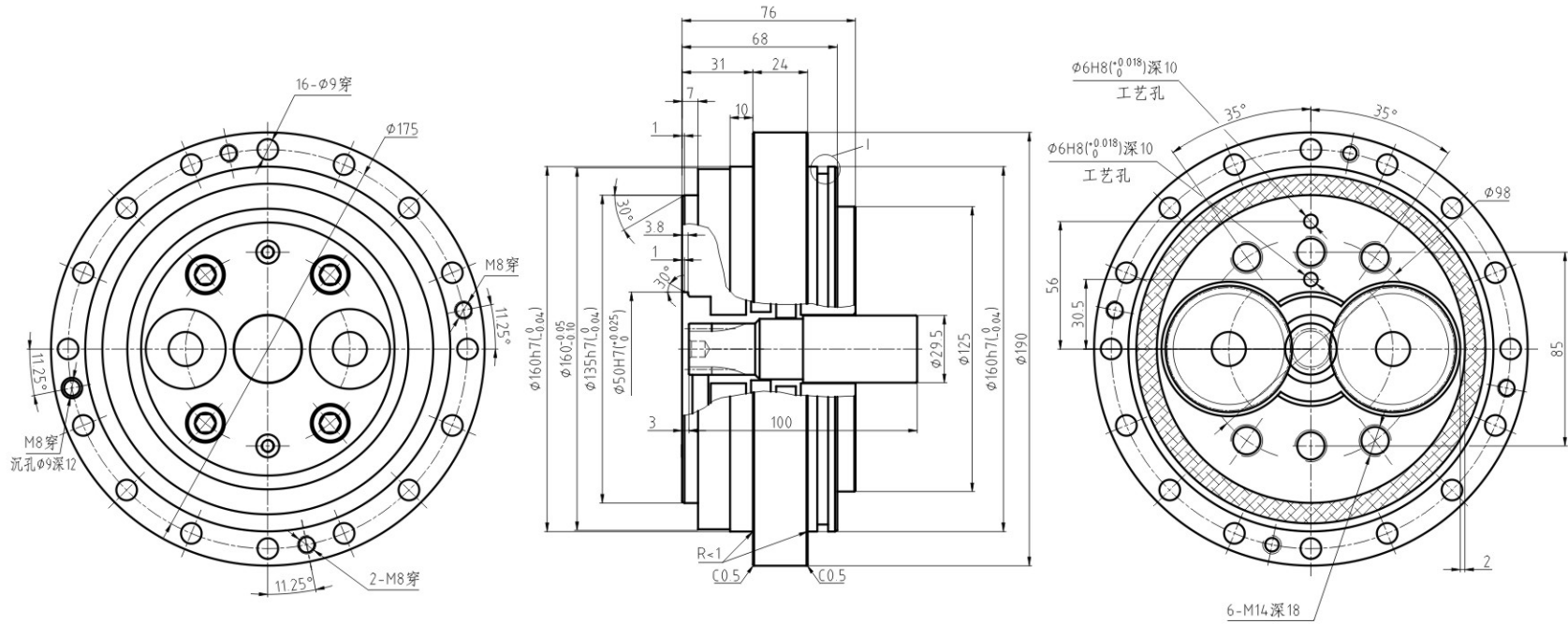
■BX40E ( 速比 : 81,105,121,153 ) 输出轴螺栓紧固型外形尺寸图
