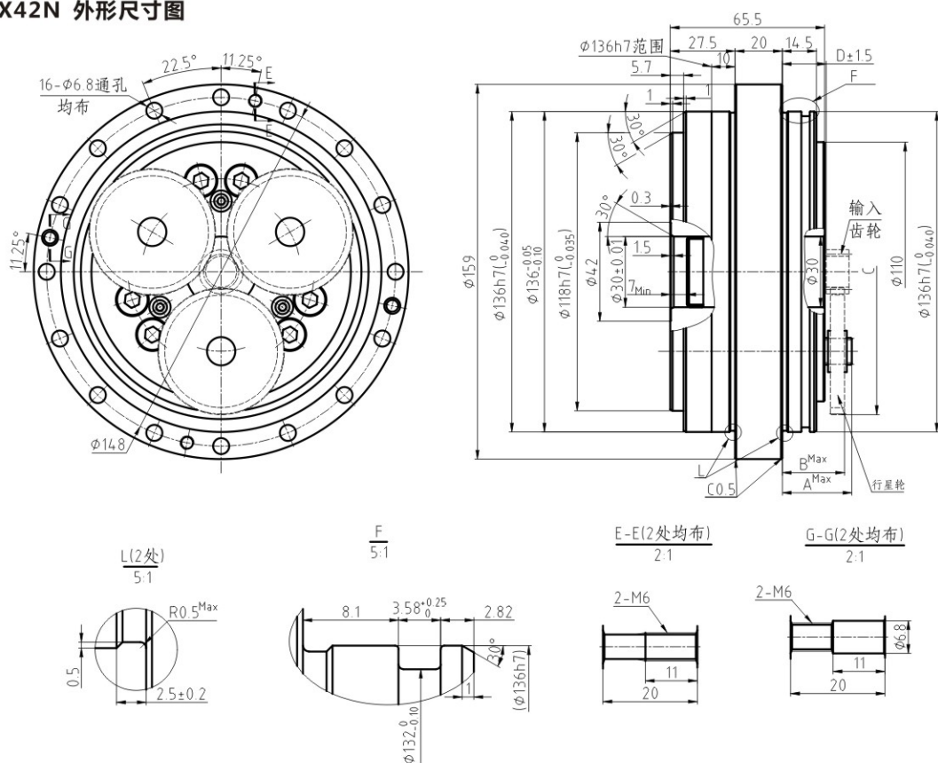
■ BX42N 外形尺寸图
