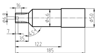
输入齿轮 型式B
