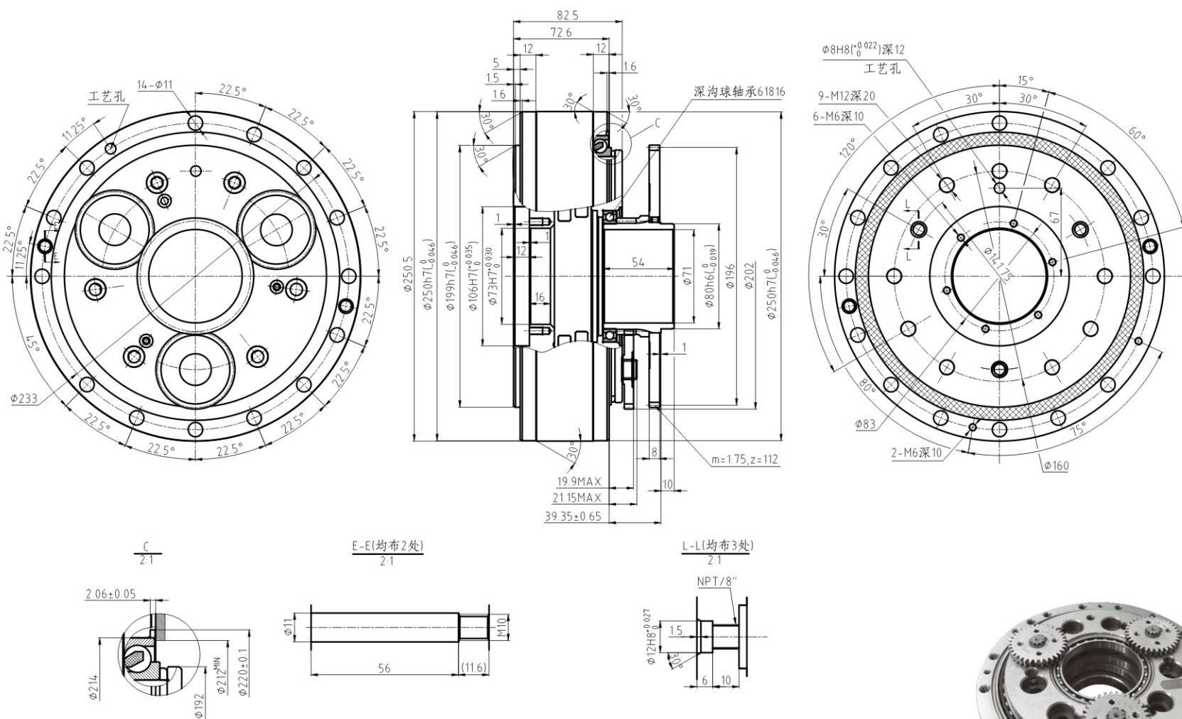
■ BX100C 输出轴螺栓紧固型外形尺寸图
