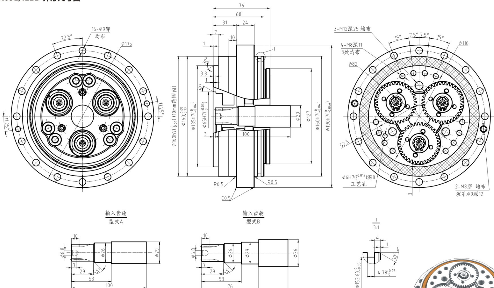
■ BX65E/i121 外形尺寸图
