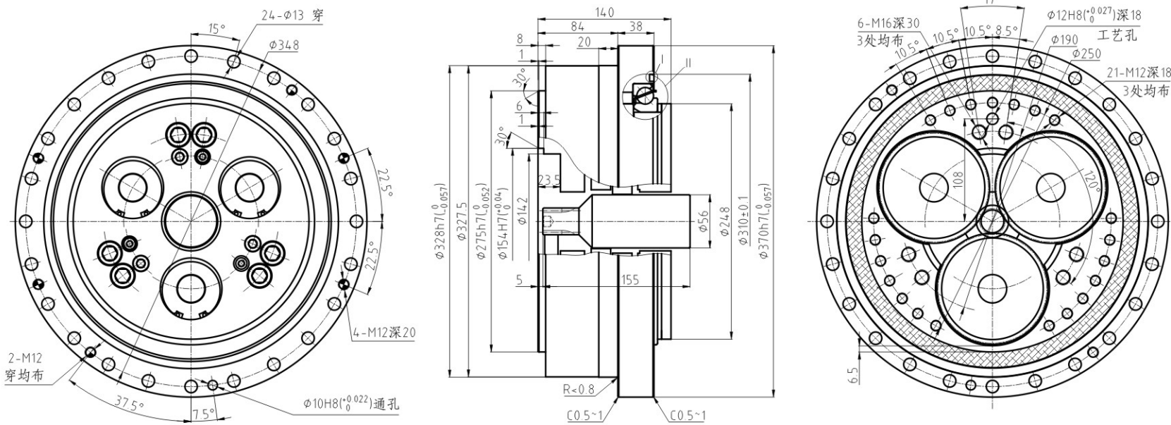
■BX450E 输出轴螺栓紧固型外形尺寸图
