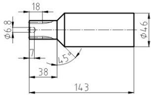
输入齿轮 型式A
