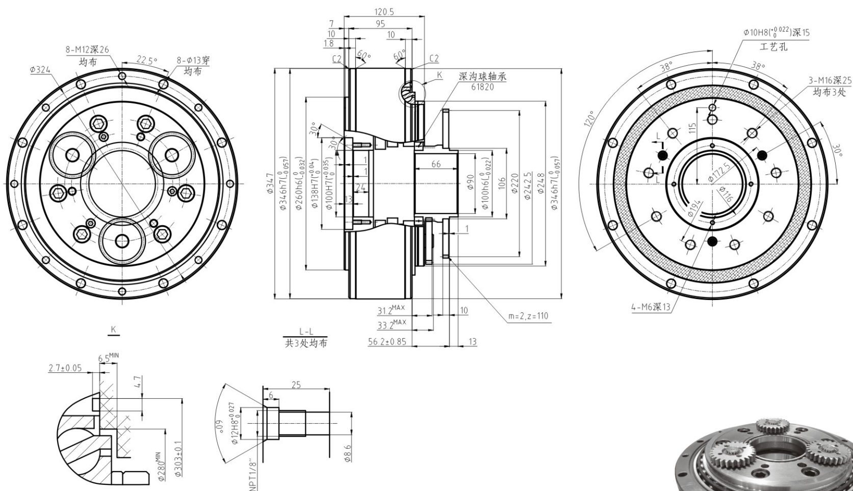
■ BX200C 输出轴螺栓紧固型外形尺寸图
