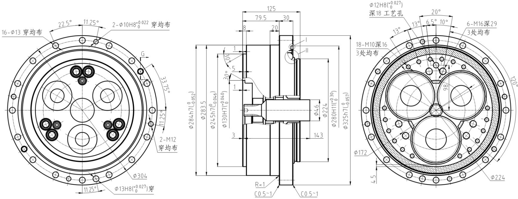
■BX320E3 输出轴螺栓紧固型外形尺寸图
