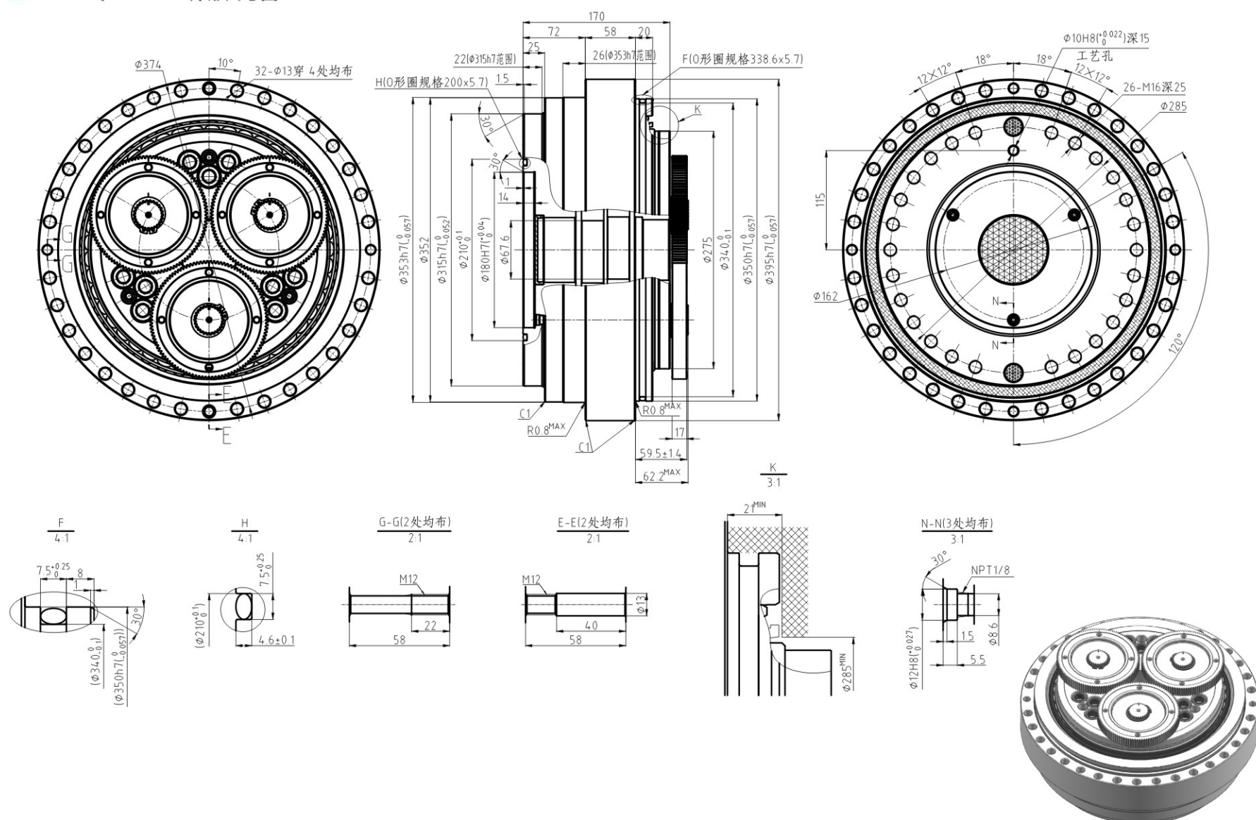
■ BX700N/i268.42 外形尺寸图
