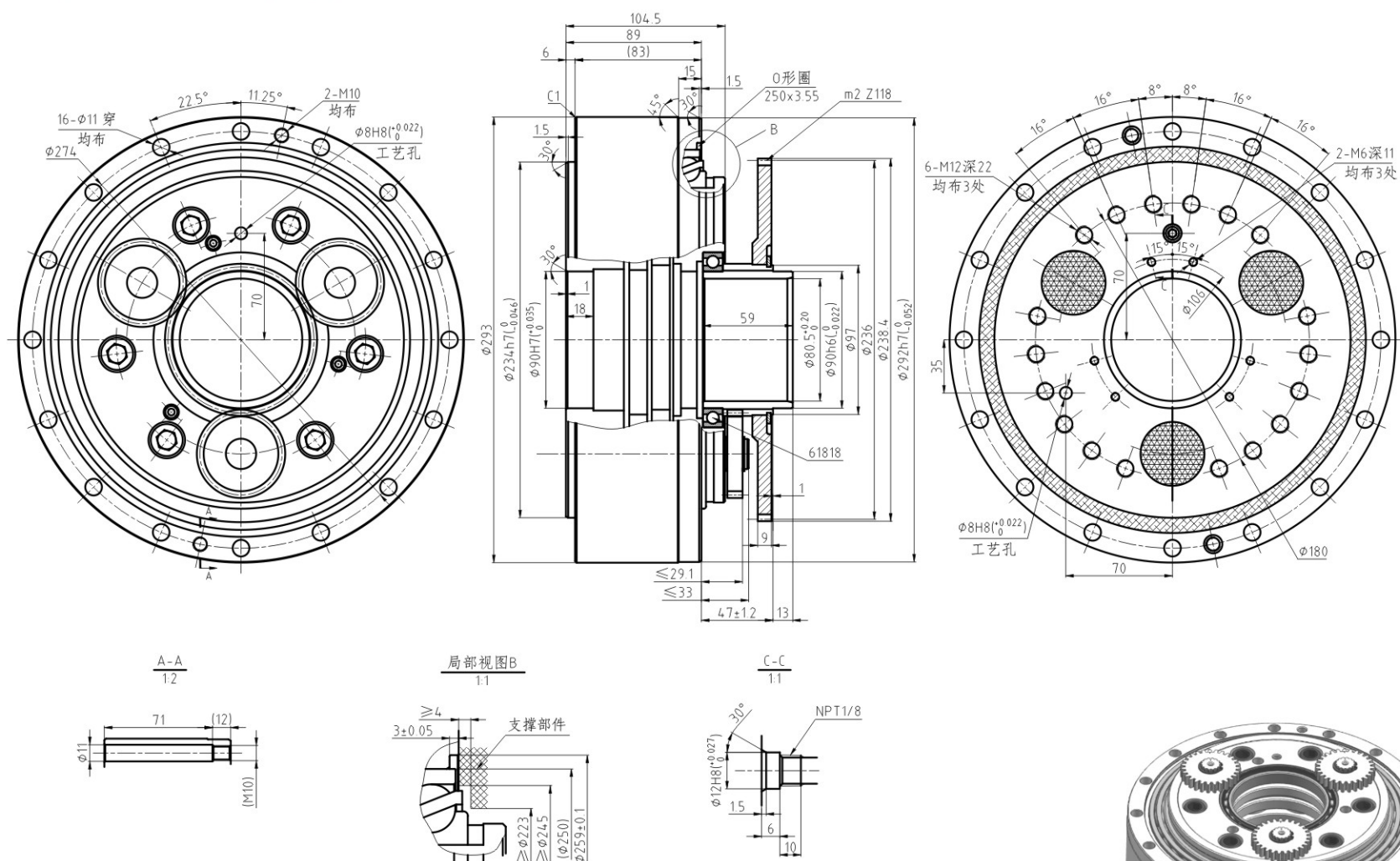
■ BX155C 输出轴螺栓紧固型外形尺寸图
