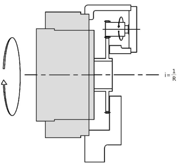
针齿壳固定行星架输出的情况
