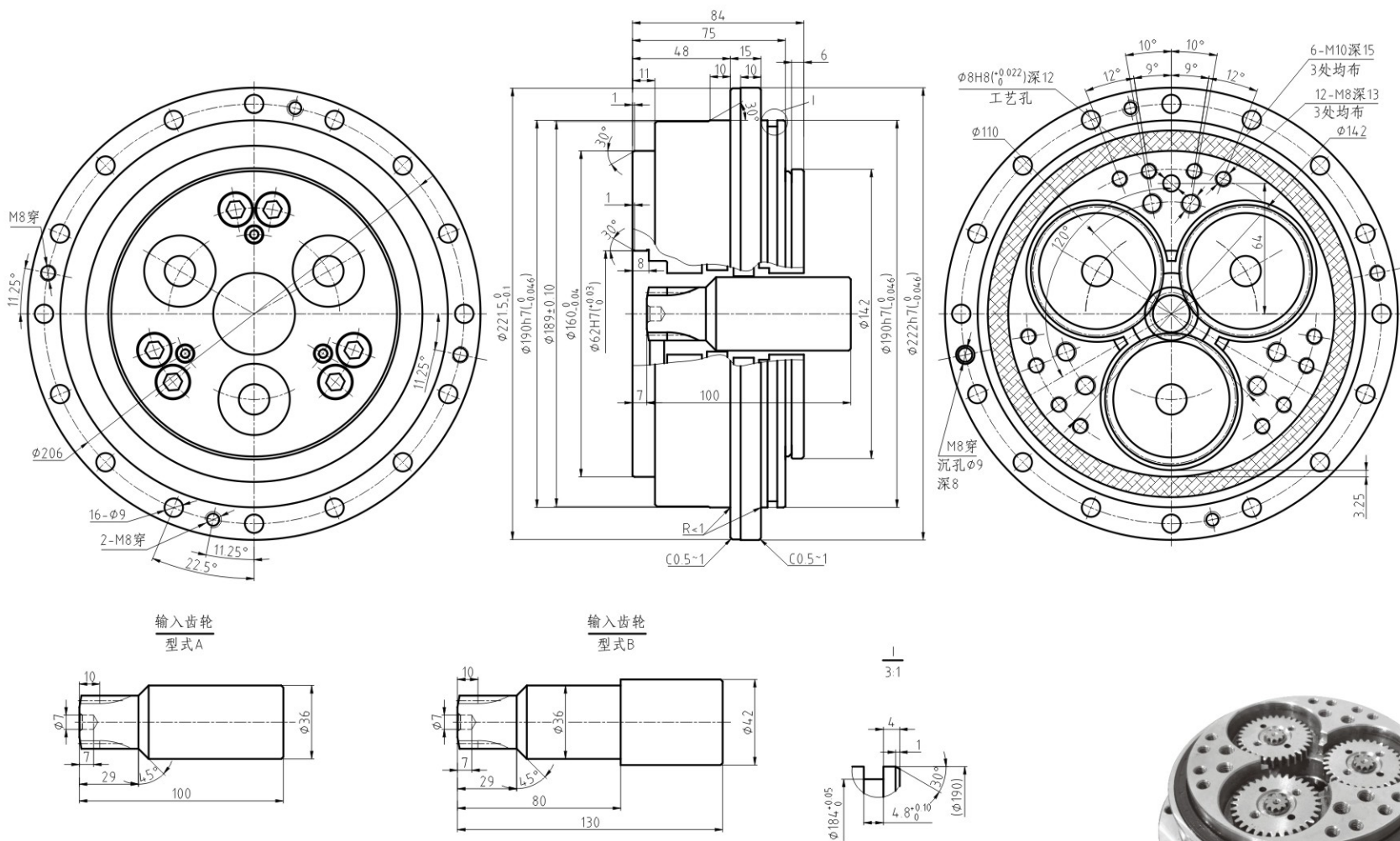
■ BX80E (速比: 81, 101, 121, 153) 输出轴螺栓紧固型外形尺寸图
