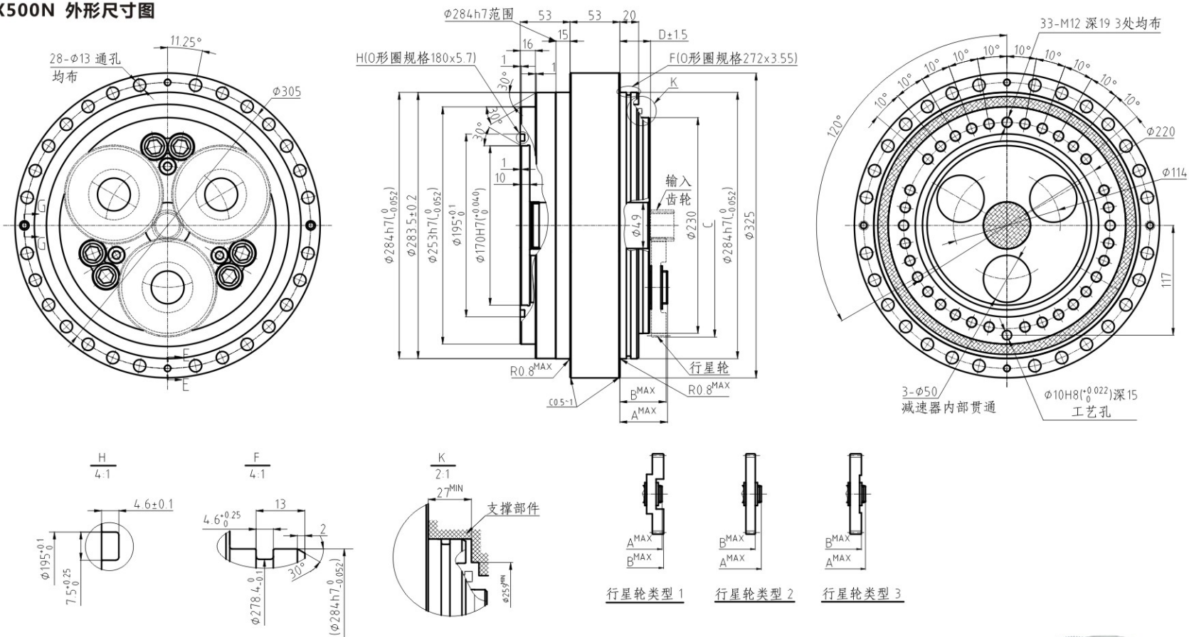
BX500N 外形尺寸图
