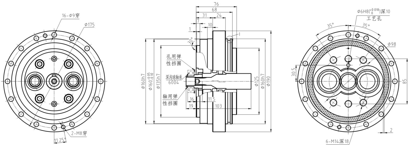
■BX40E/i57 输出轴螺栓紧固型外形尺寸图
