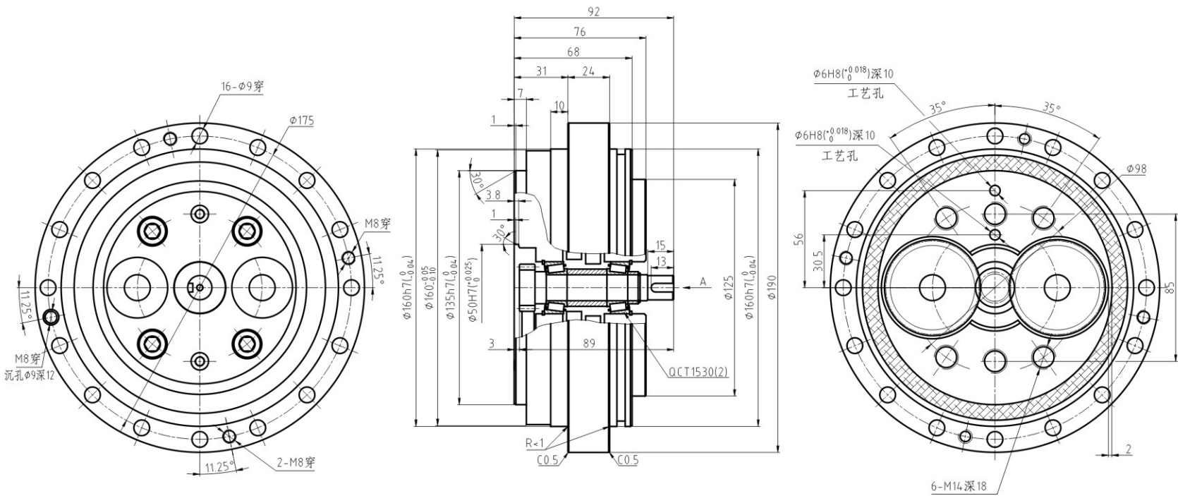
■BX40E/i81S 外形尺寸图
