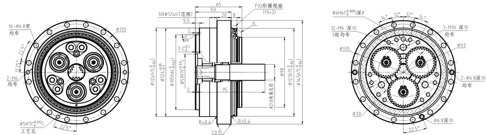
■BX35E/i121 外形尺寸图
