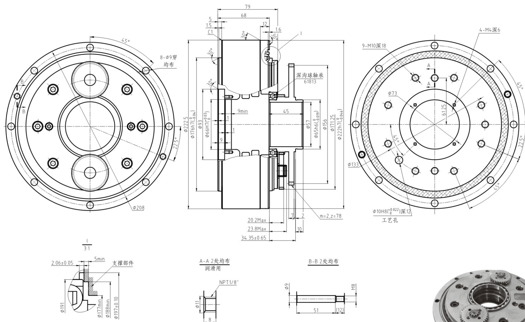
■ BX50C 输出轴螺栓紧固型外形尺寸图
