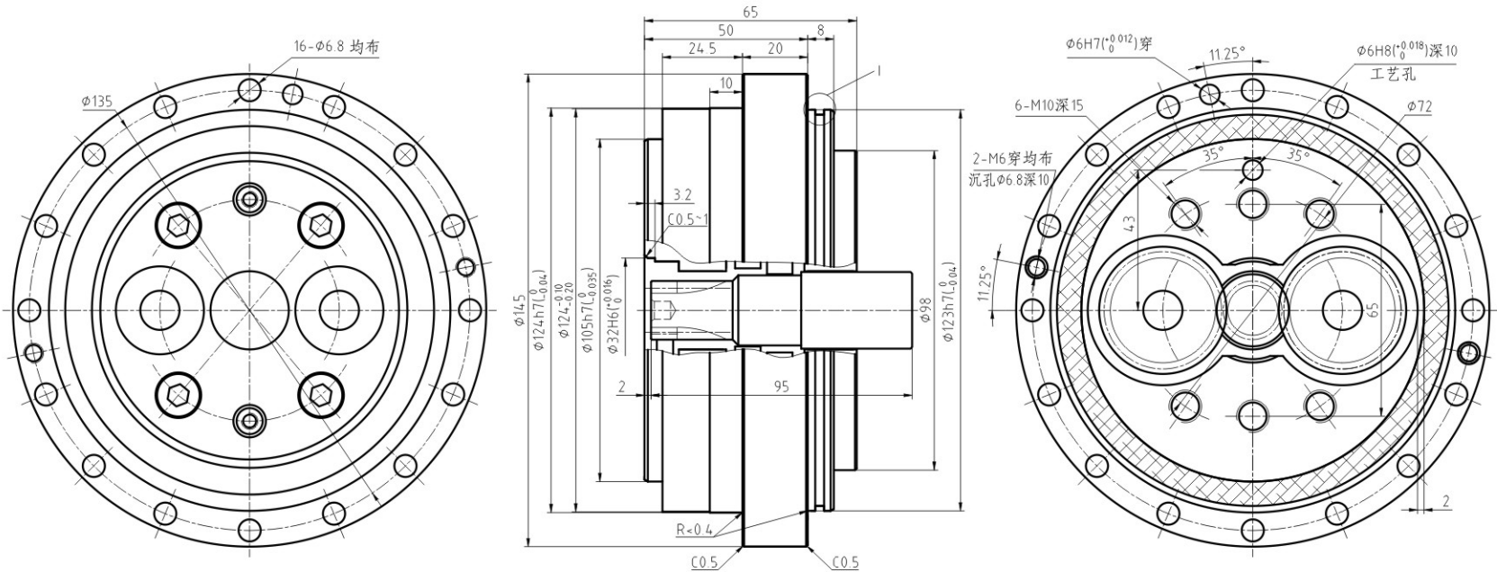
■BX20E ( 速比：81,105,121,141,161 ) 输出轴螺栓紧固型外形尺寸图 型号：BX20E- □ ( 速比 ) - A B
