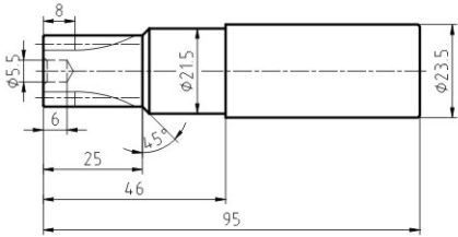
输入齿轮 型式A
