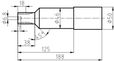
输入齿轮 型式B
