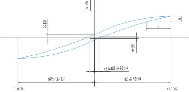
迟滞曲线
