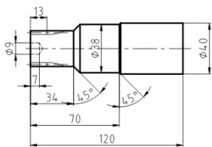
输入齿轮 标准型式
