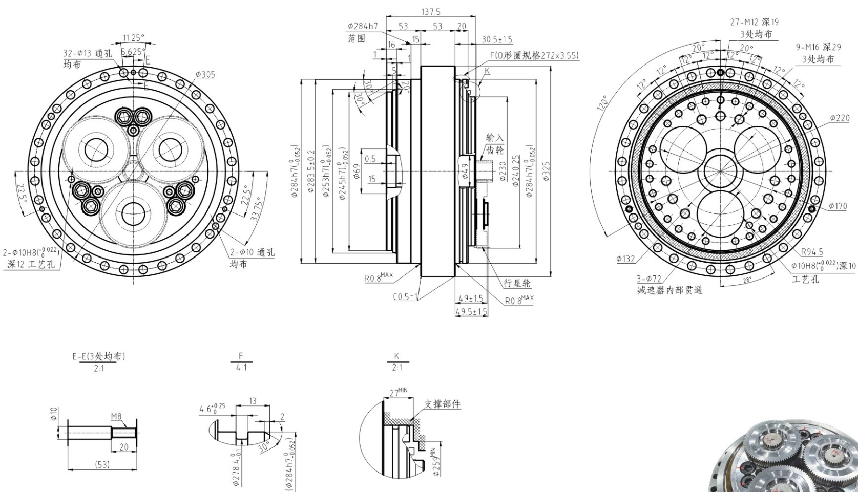
■BX500N/i222T 外形尺寸图
