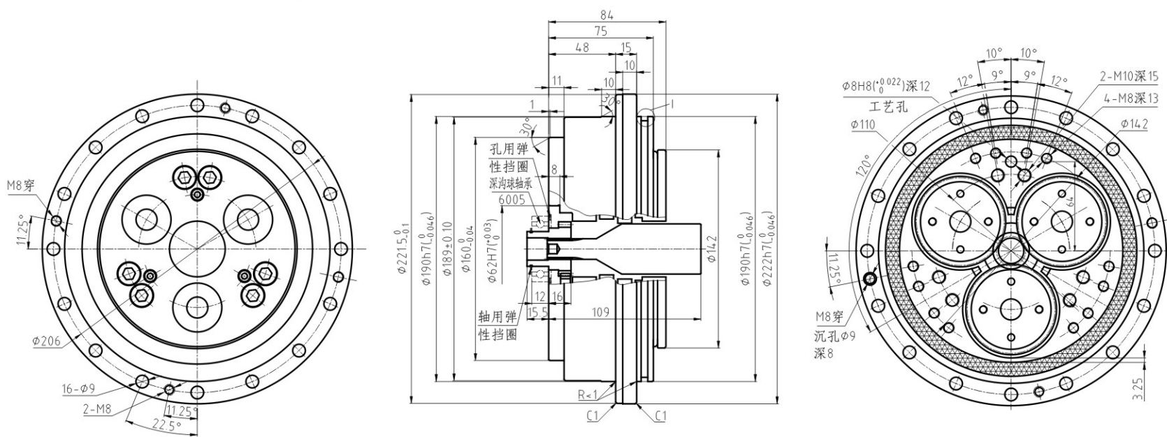
■ BX80E/i57 输出轴螺栓紧固型外形尺寸图
