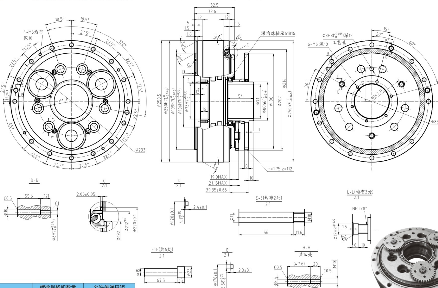
■ BX120C 输出轴通孔螺栓紧固型外形尺寸图
