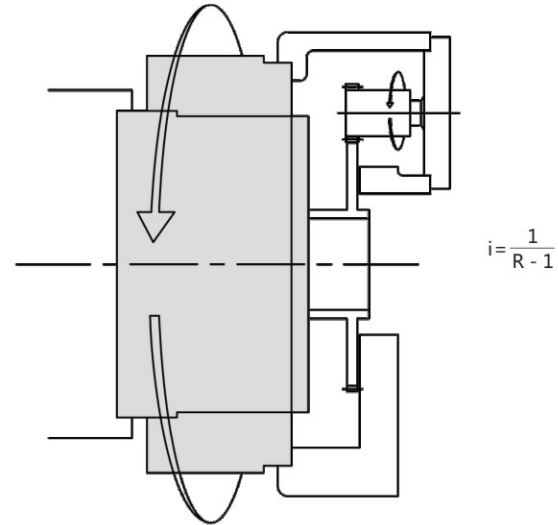
行星架固定针齿壳输出的情况
