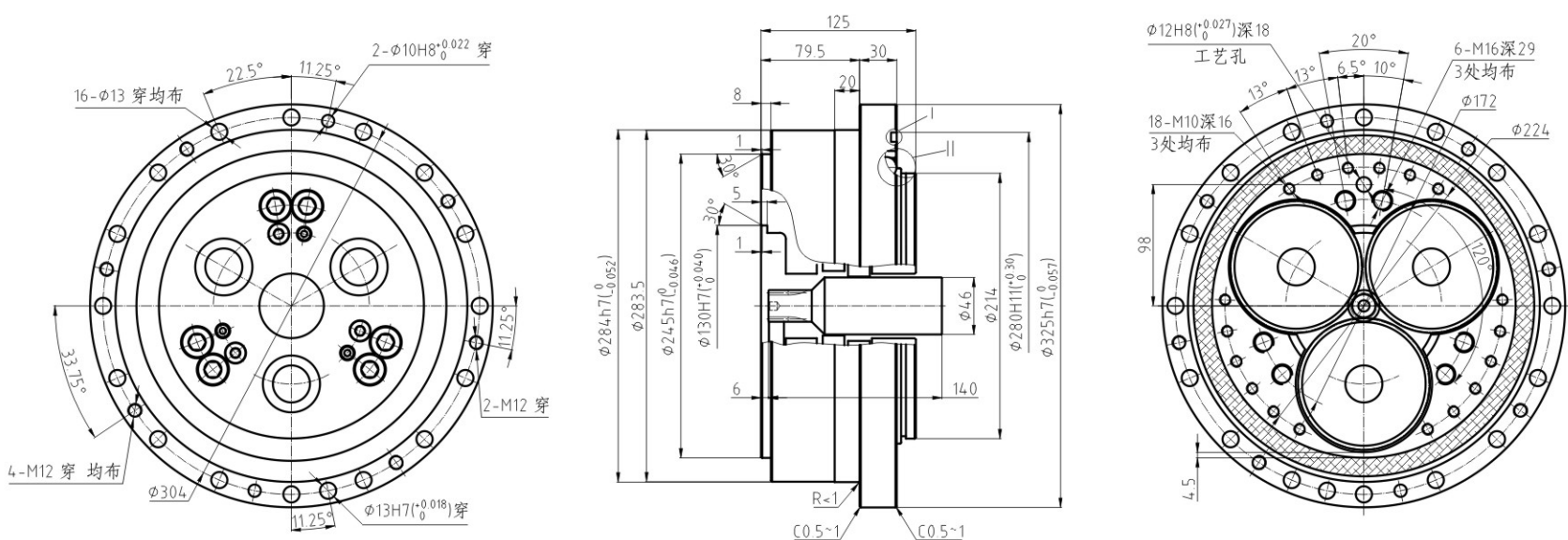
■ BX320E 输出轴螺栓紧固型外形尺寸图
