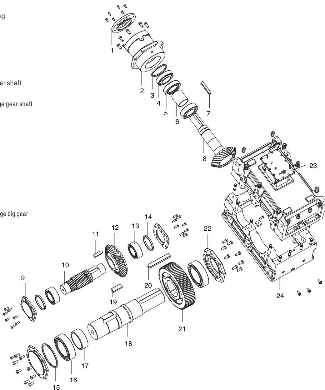
B系列结构图:/ B series structure drawing:
